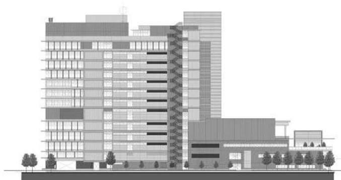
北立面图
