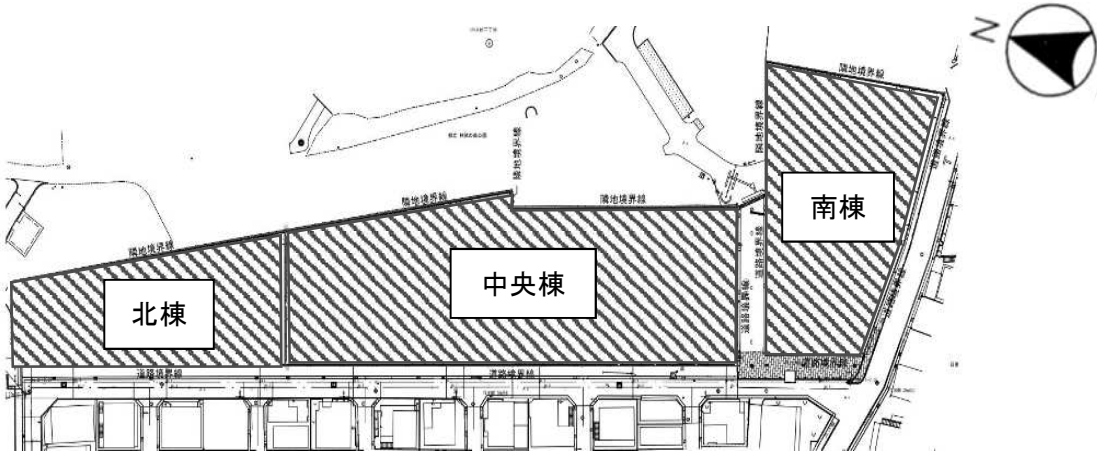
配置図
