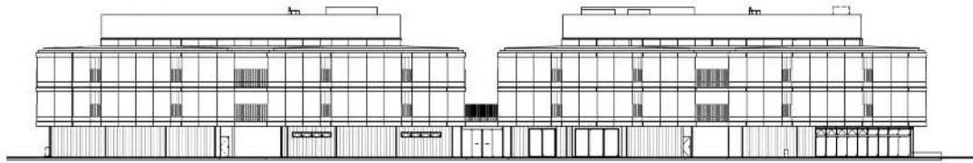
西立面图
