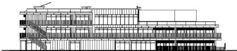
東立面图
