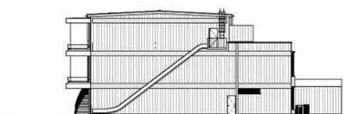
東立面图
