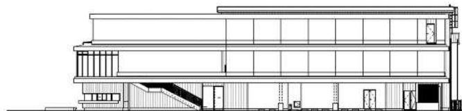
南立面图
