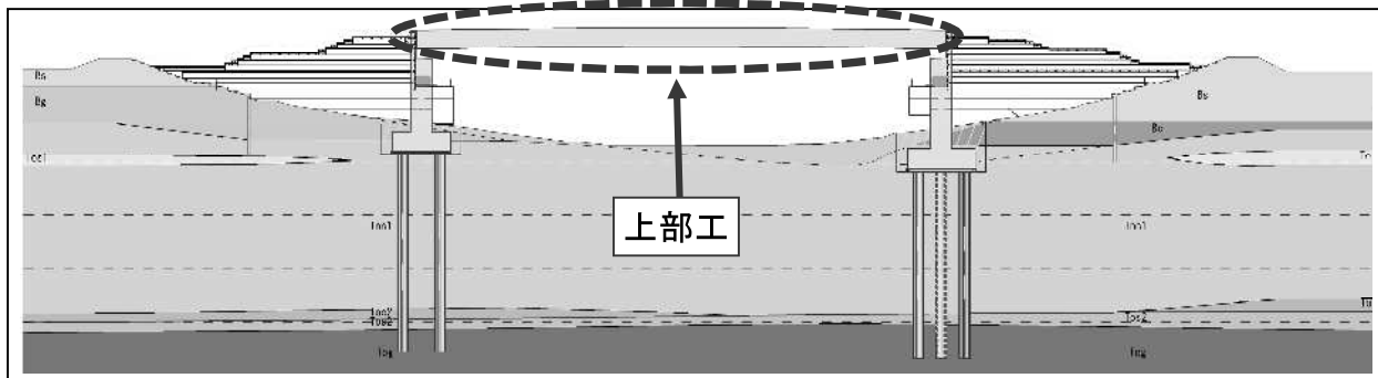
断面図
