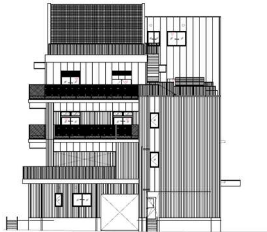
東立面图
