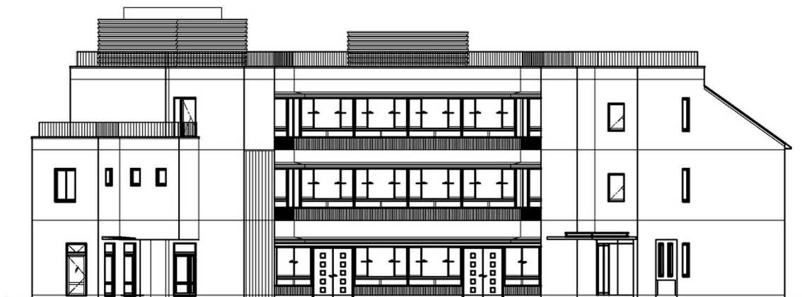
南東立面图
