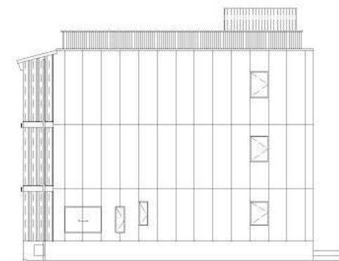
北東立面图
