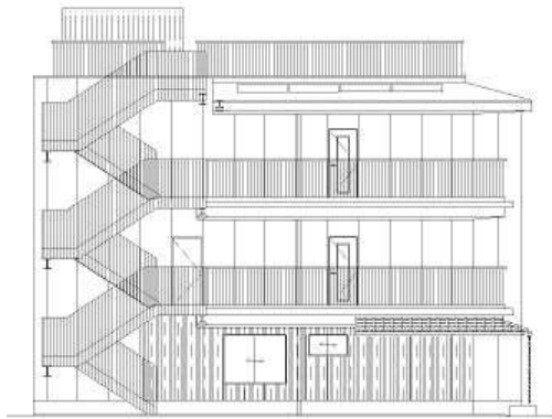
南西立面图
