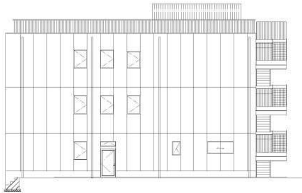
北西立面图
