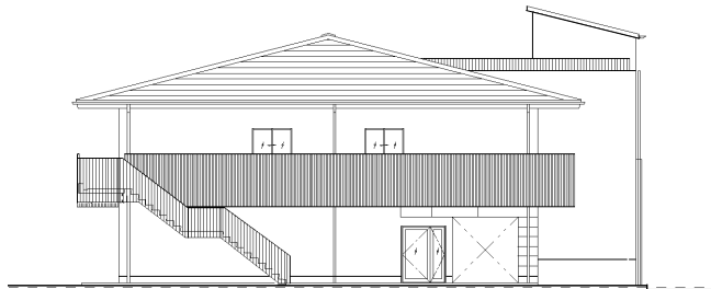
北立面图
