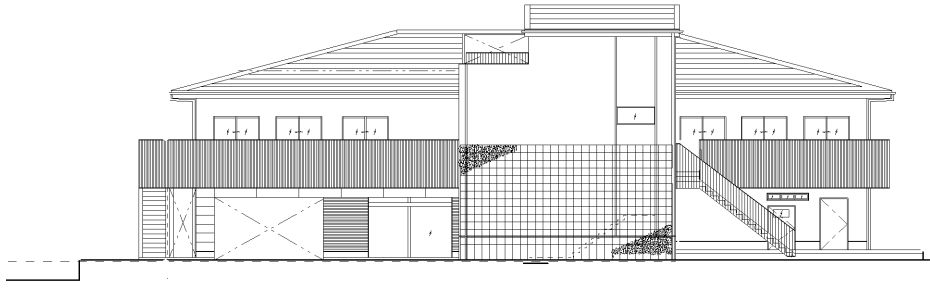
西立面图
