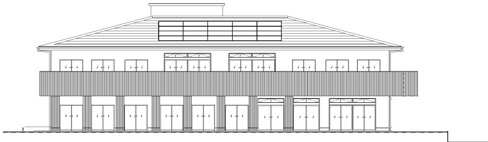
東立面图
