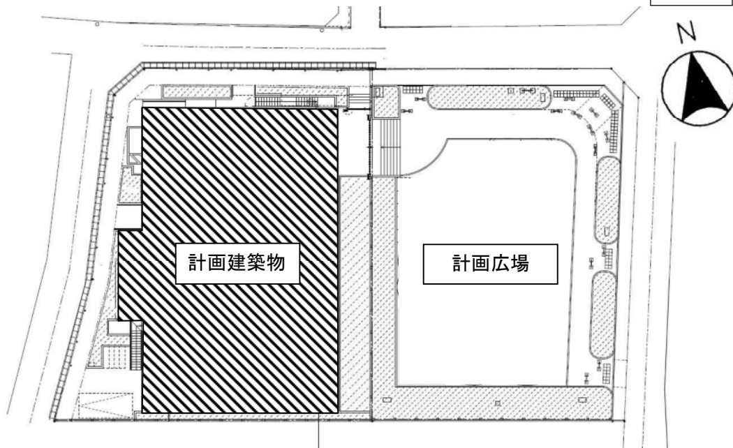
配置図
