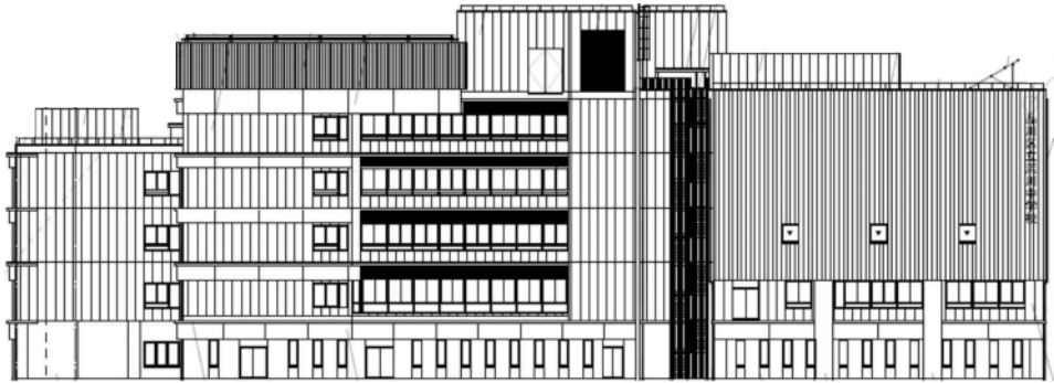
東立面图
