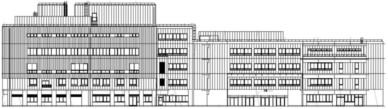
北立面图
