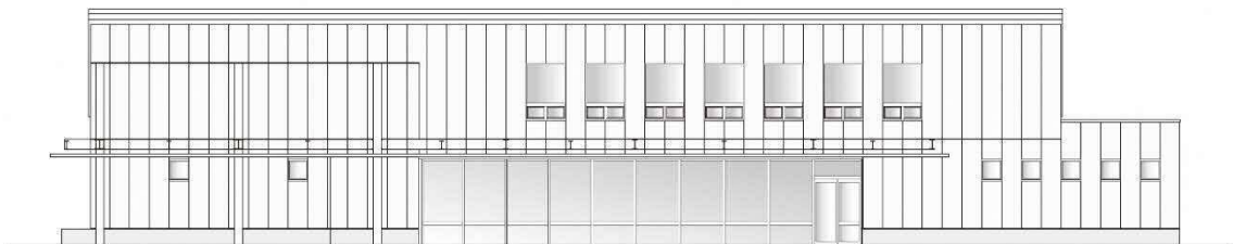
東立面图
