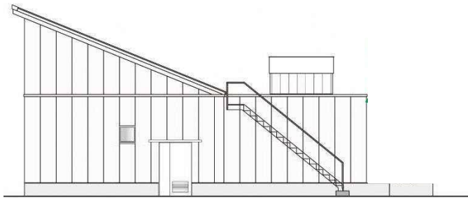
北立面图
