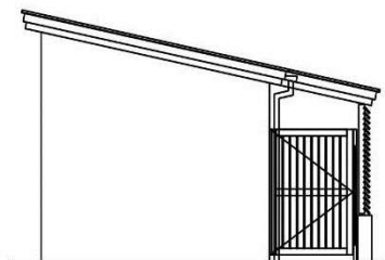
北立面图
