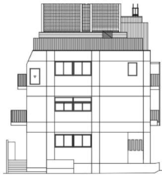
西立面图
