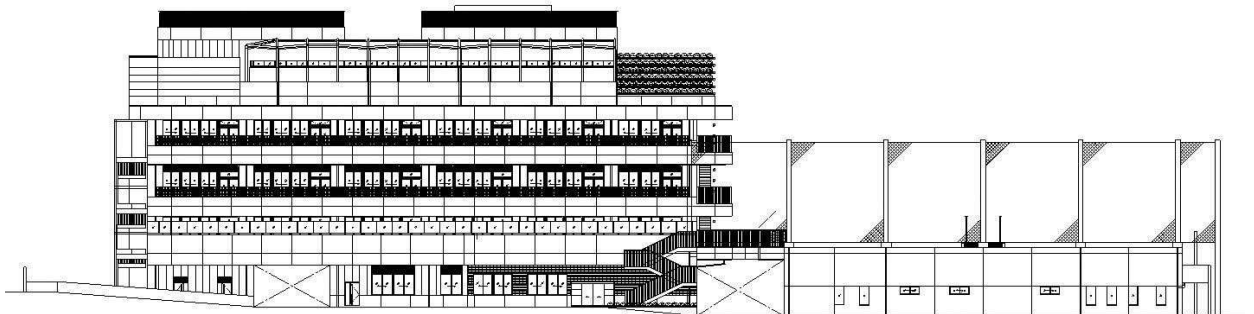
南東立面图
