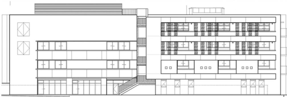
南立面图
