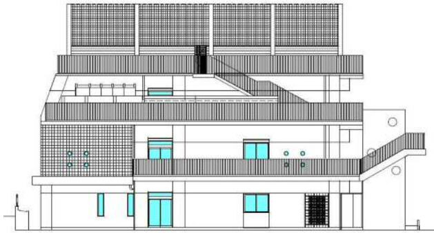
北立面图
