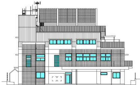
東立面图
