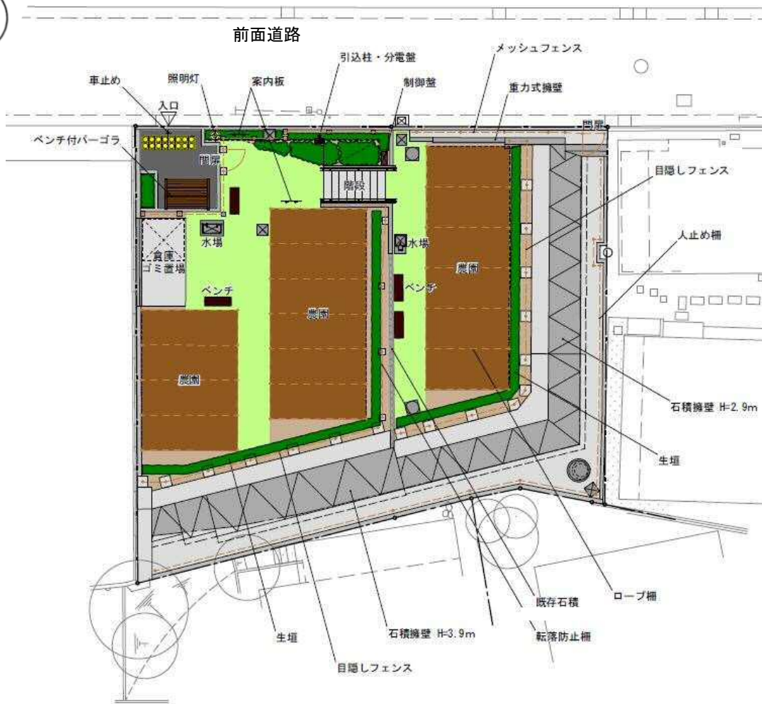
計画平面図
