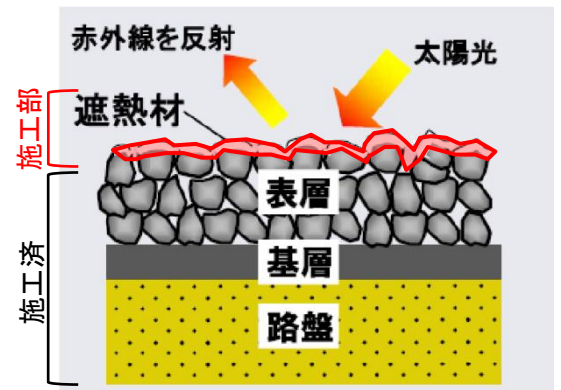
【舗装断面イメージ図】 出典：国土交通省ホームページ
