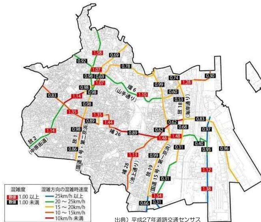
図2-14 道路混雑度と混雑時速度の状況
