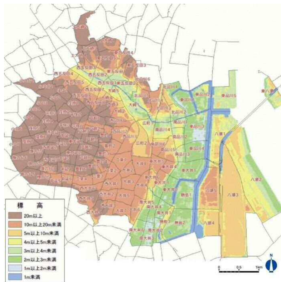
図2-16 区内の標高
