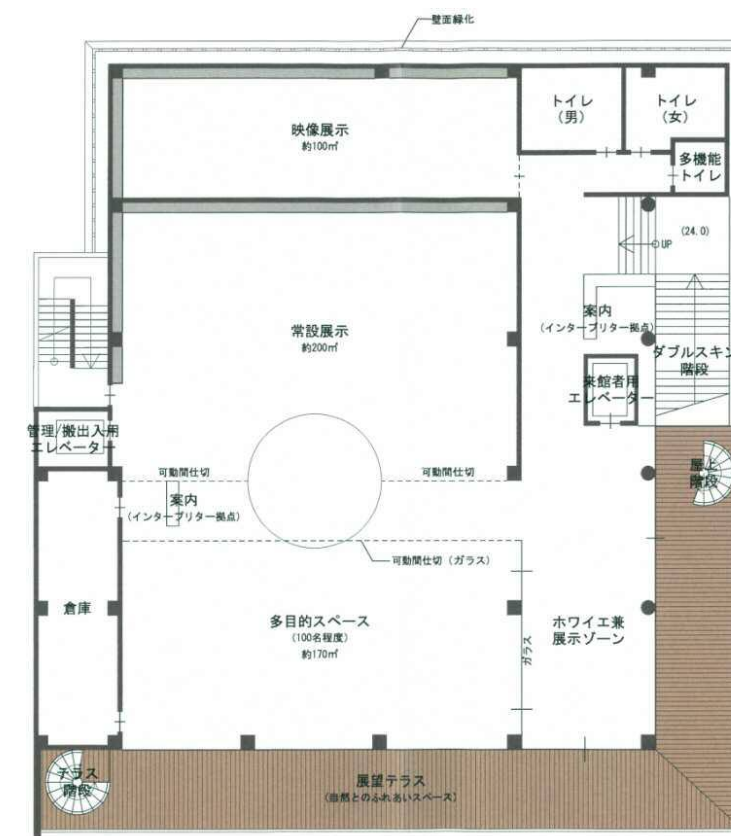
3階平面図
