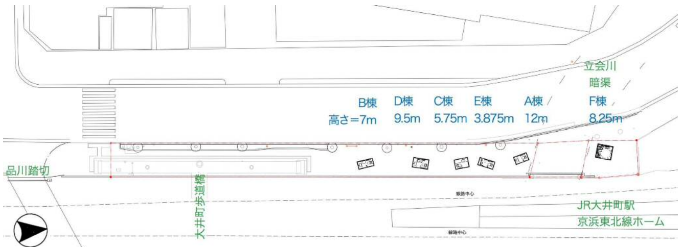
平面図
