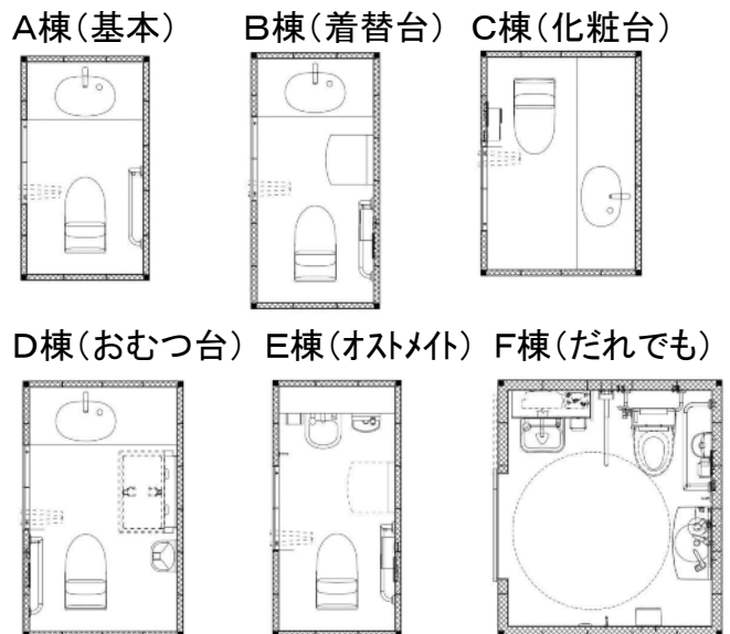
建物平面図
