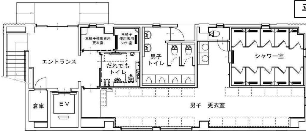
1階平面図
