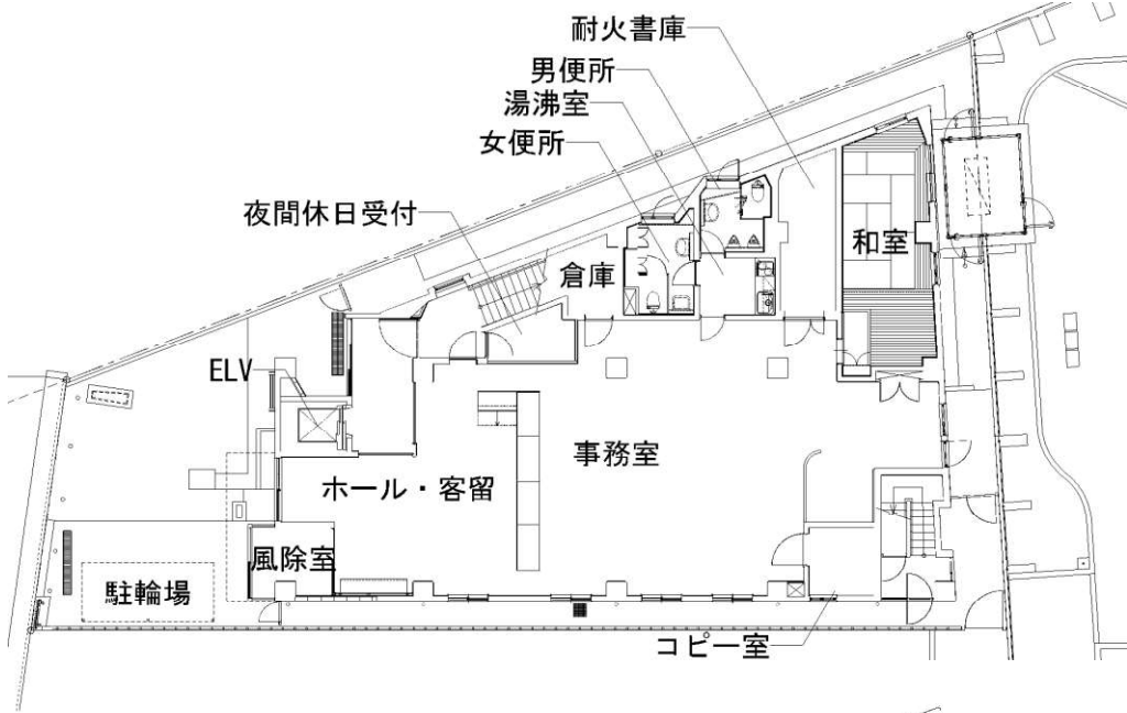
改修後 1階平面図
