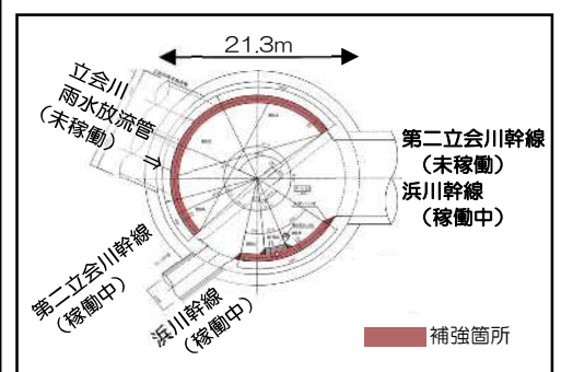
【なぎさ会館人孔補強イメージ】
