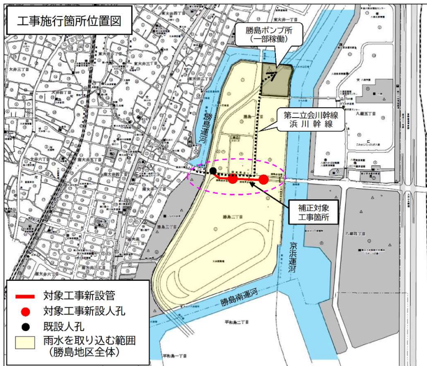
詳細図
