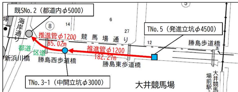
詳細図
