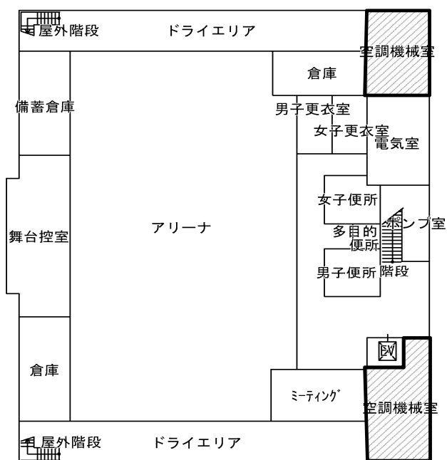
B1階平面図
