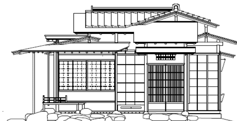
南側立面図
