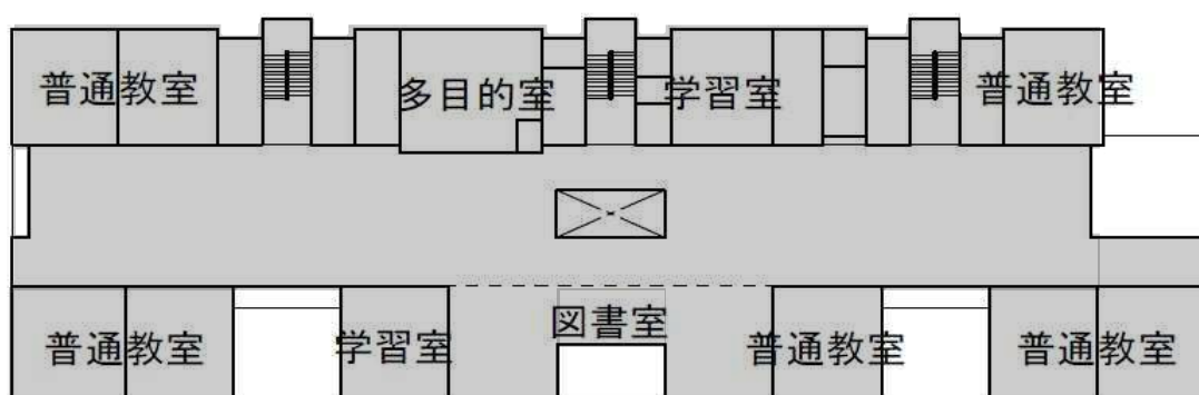
5F平面図
