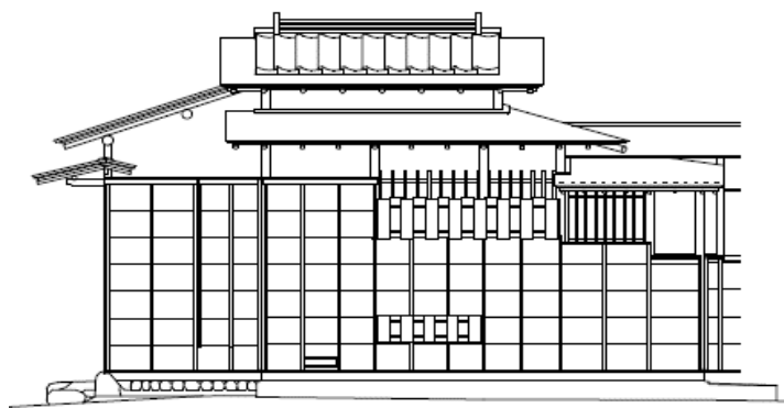
北側立面図
