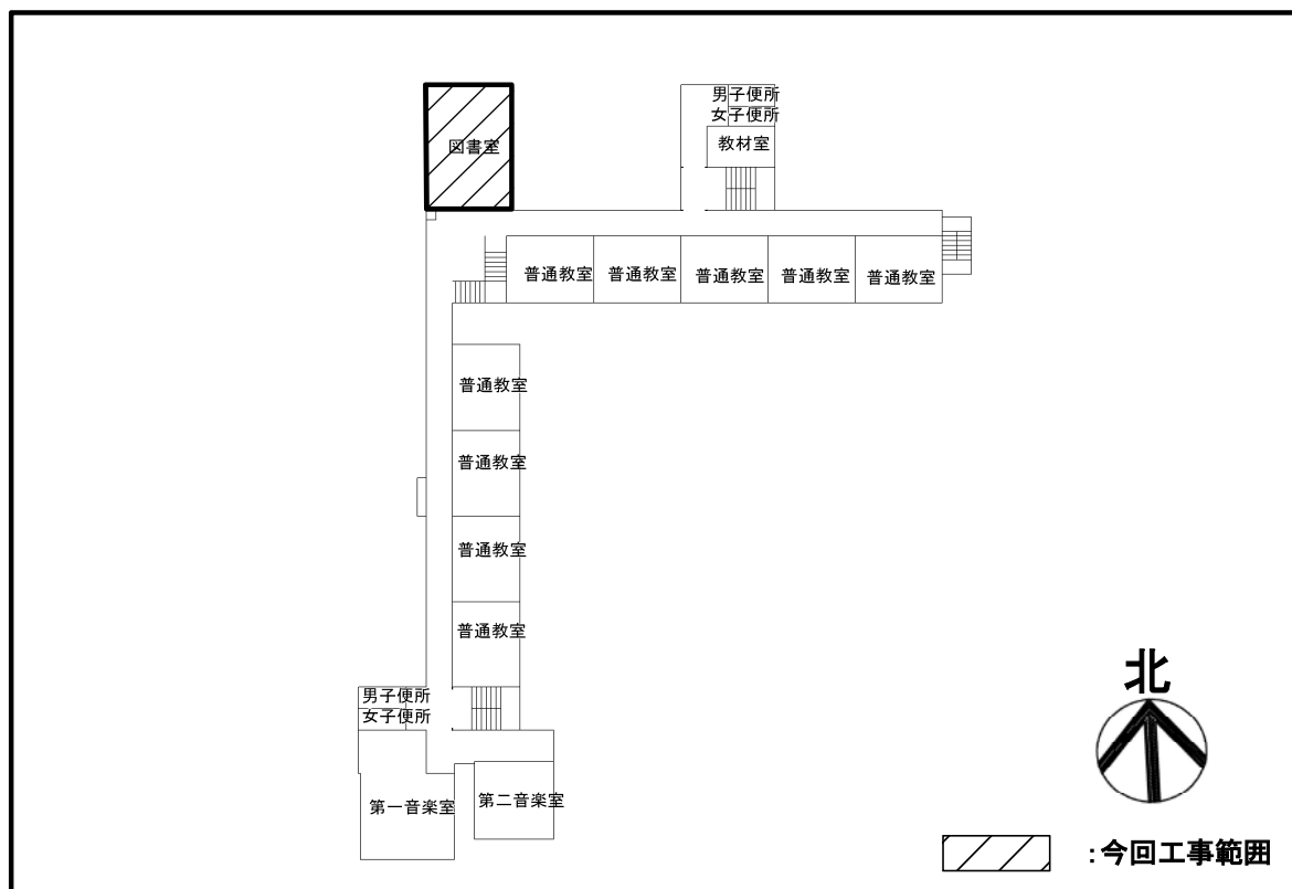
3階平面図
