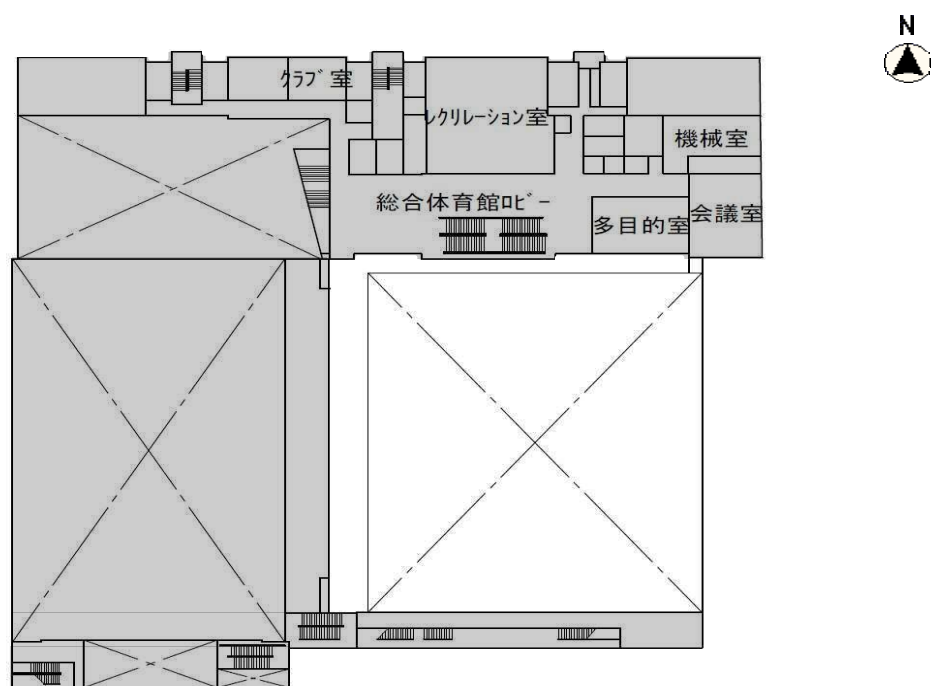
B1F平面
