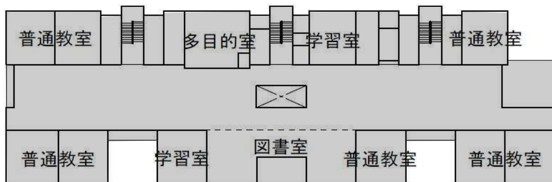
5F平面図
