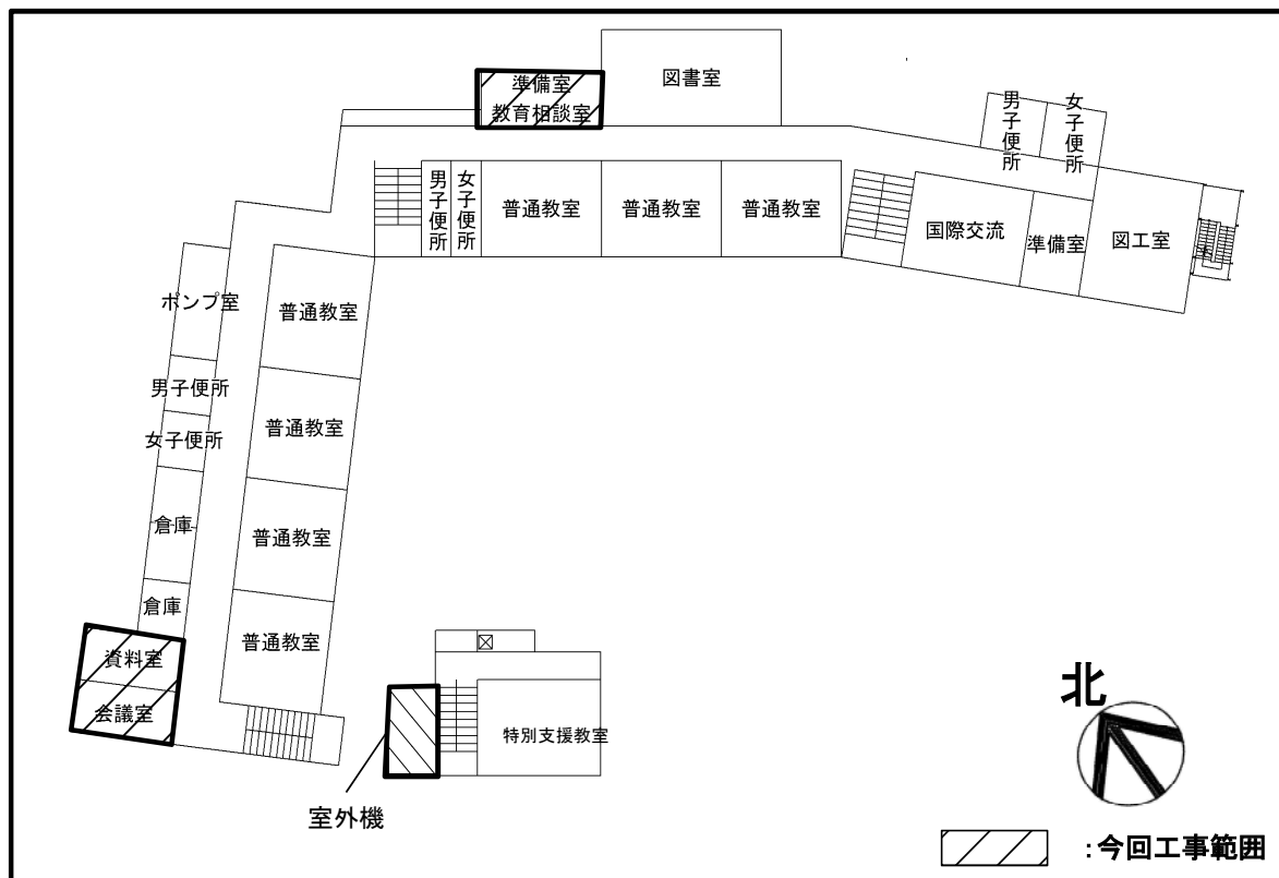
2階平面図
