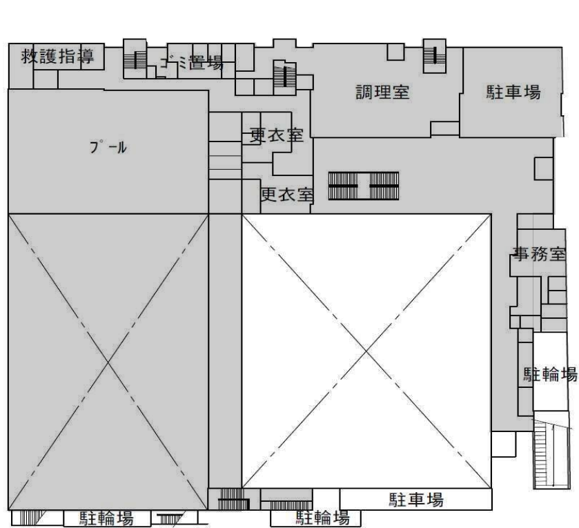
1F平面図
