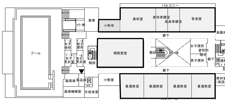
4階平面図
