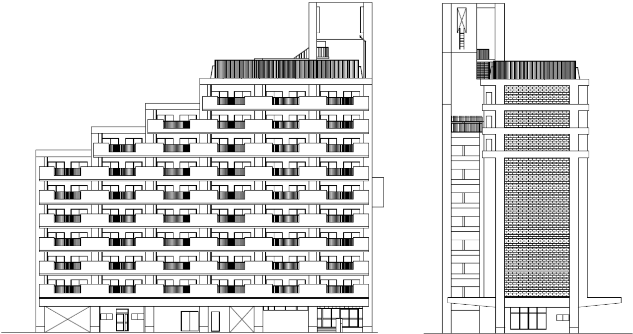
北侧立面图
