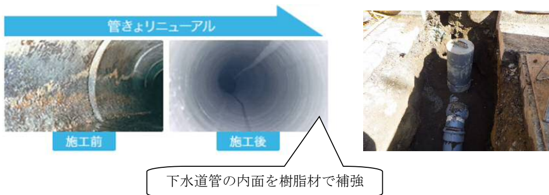
開削工法
