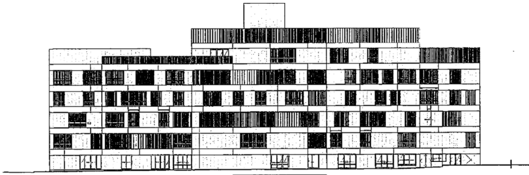
北立面图
