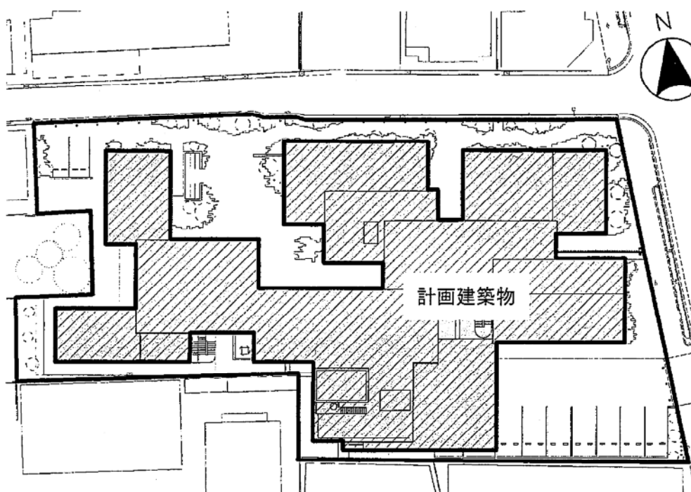
配置図
