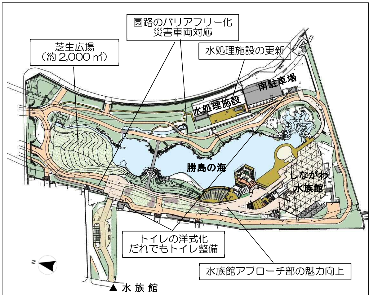
計画平面図（案）
