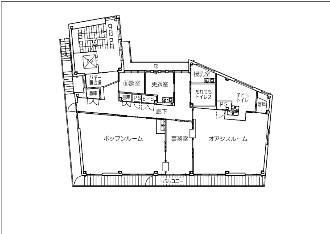
2階平面図
