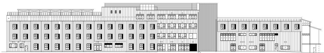
南立面図
