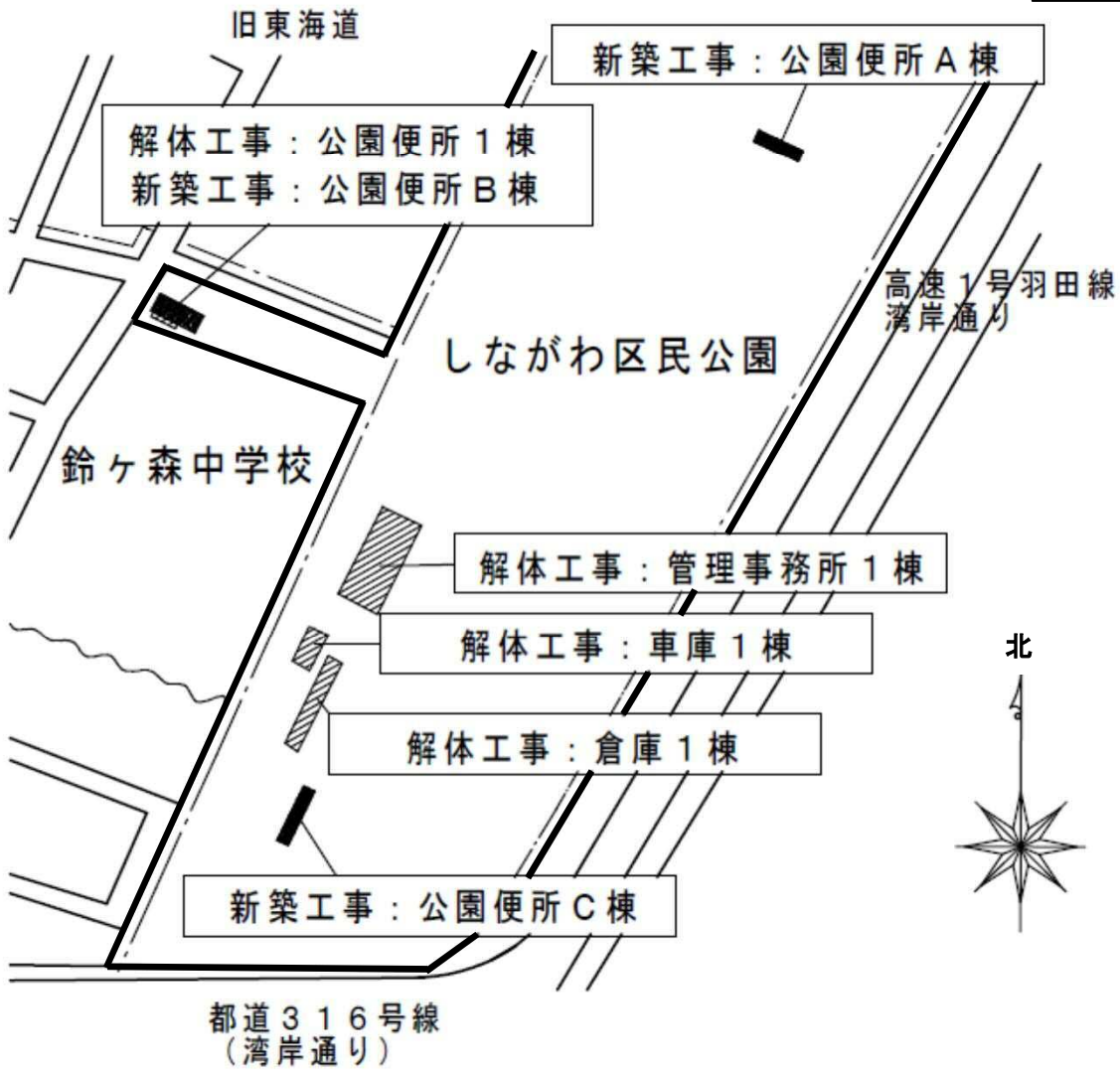
配置図
