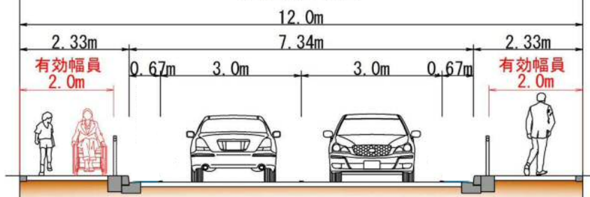
計画断面図
