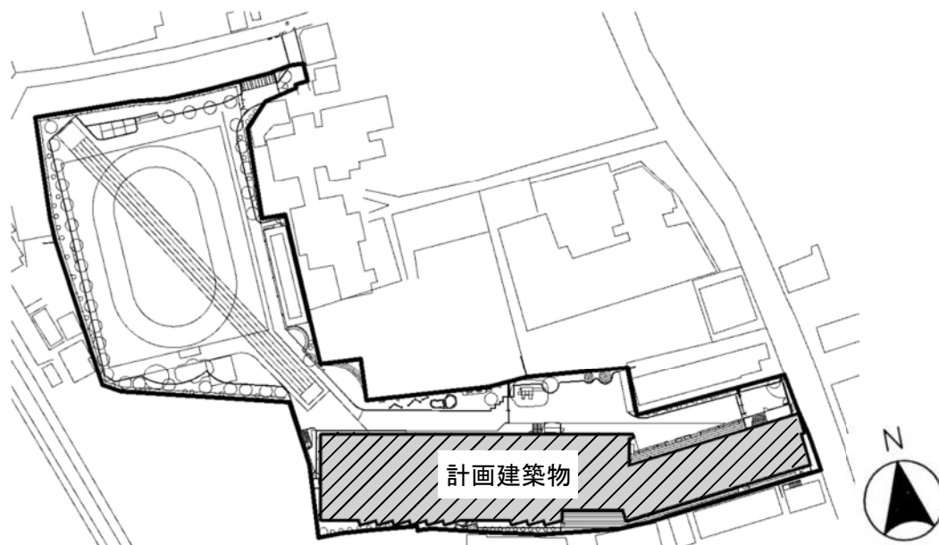
配置図
