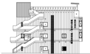
西立面图
